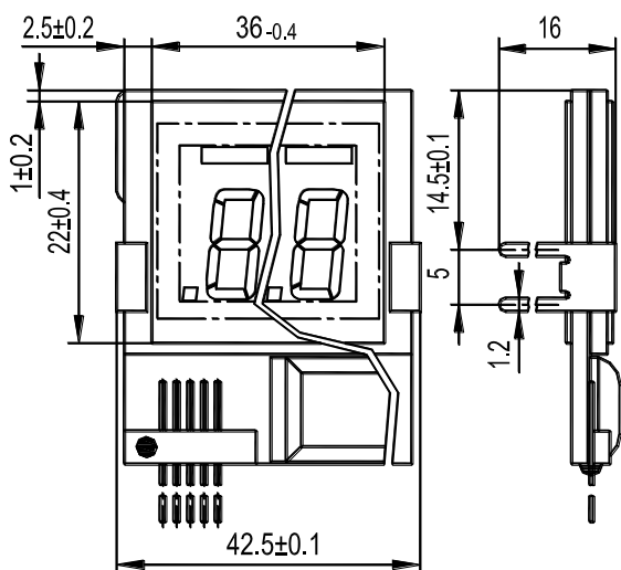
Рис.2 - ИВУ KF128Тх1хх[1-4], остальное - см. рис.1
