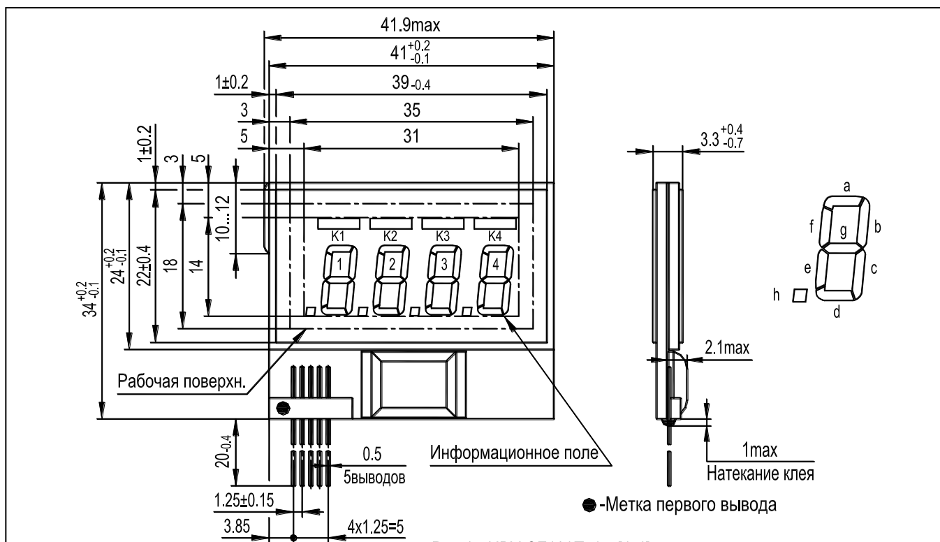
Рис.1 - ИВУ CF128Тх1хх[1-4]
