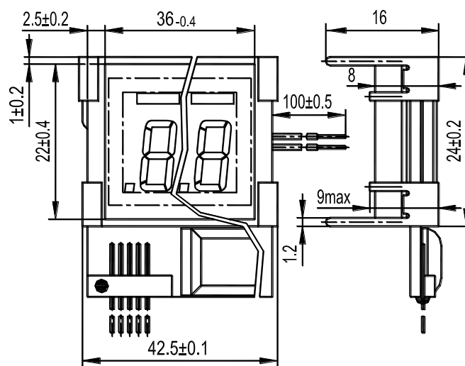
Рис.3 - ИВУ KF128Тх1хх[1-4]-Dx, остальное - см. рис.1
