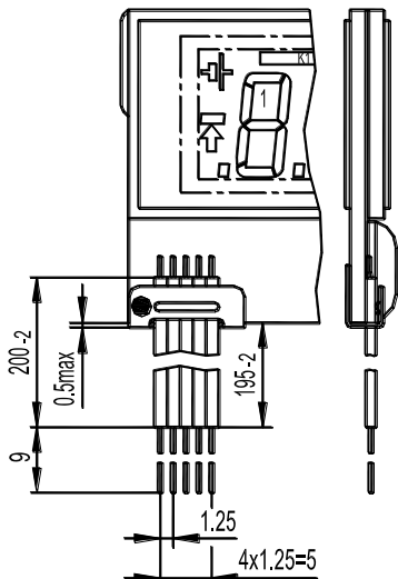
Рис.2 - ИВУ CS153Tх3xx[2,4,7,9], остальное - см. рис.1
