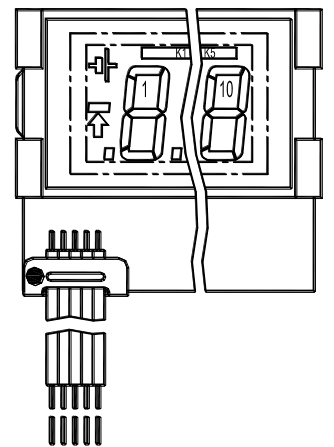
Рис.4 - ИВУ KS153Tх3xx[2,4,7,9], остальное - см. рис.1, 2, 3
