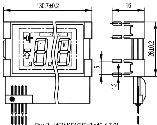
Рис.3 - ИВУ KF153Tх3xx[2,4,7,9], остальное - см. рис.1
