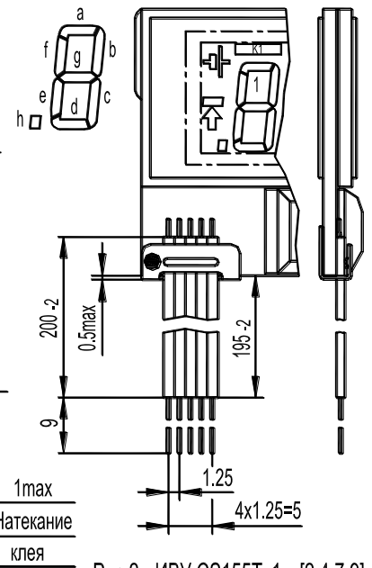
Рис.2 - ИВУ CS155Tx1xx[2,4,7,9], остальное - см. рис.1
